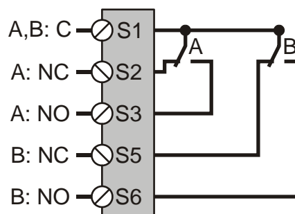
Fig. 14. End switches (Nxx-SW2)
